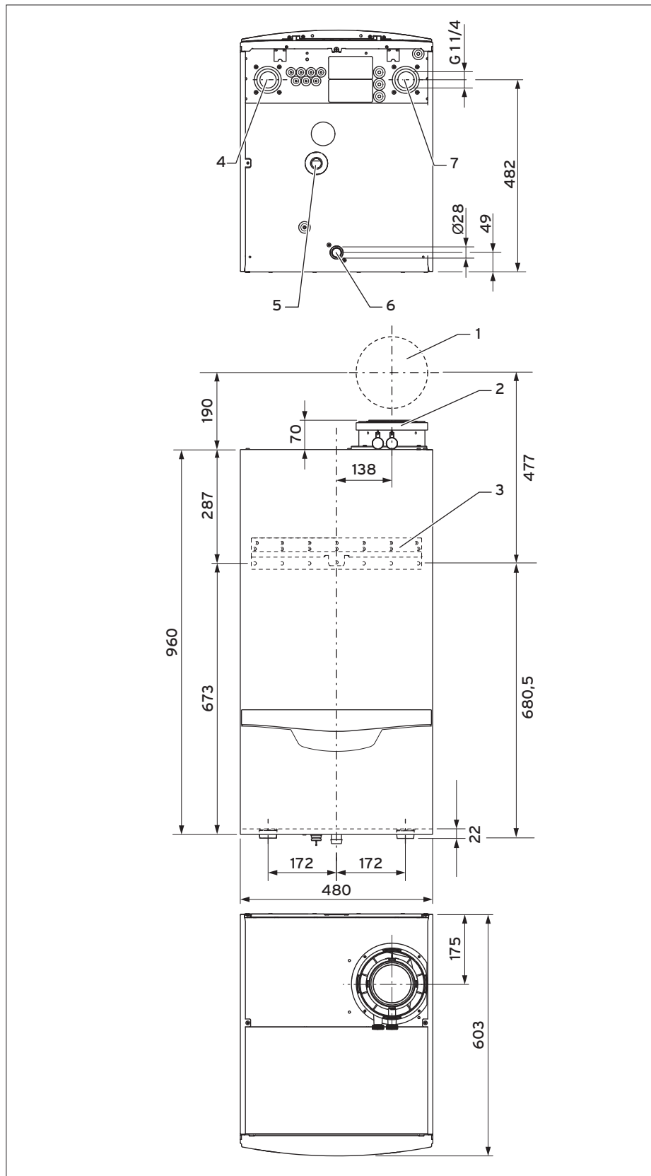
Schéma s rozměry a přípojovací míry
